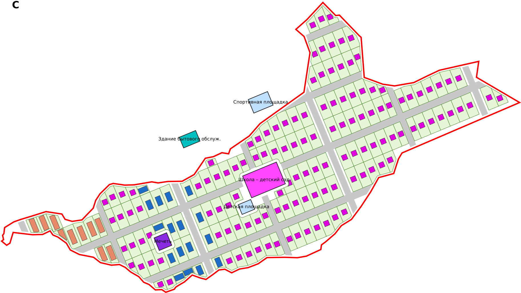
Схема планировочной организации земельного участка. М 1:2000
